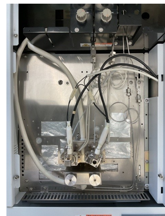
【注入口と検出器(FID)】
