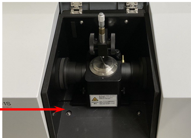
【ATR装置-設置状態】
