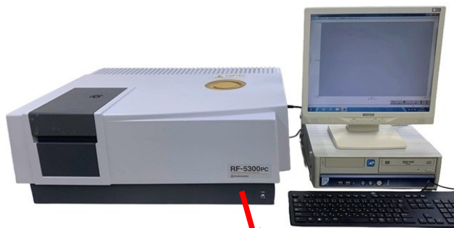
【装置全景】
