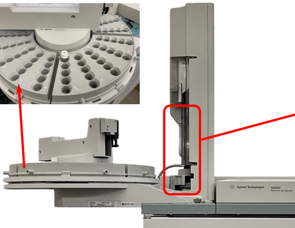
【オートサンプラー全景およびトレイ拡大】
