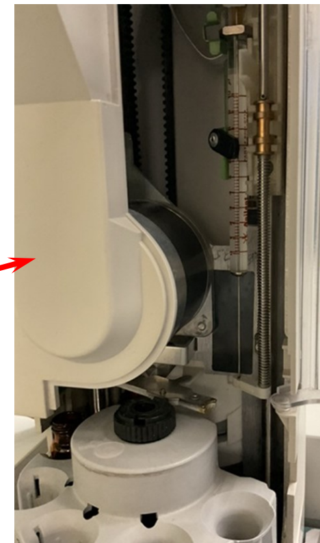
【オートインジェクター-拡大】
