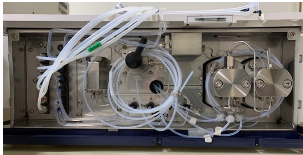
【ポンプ】
