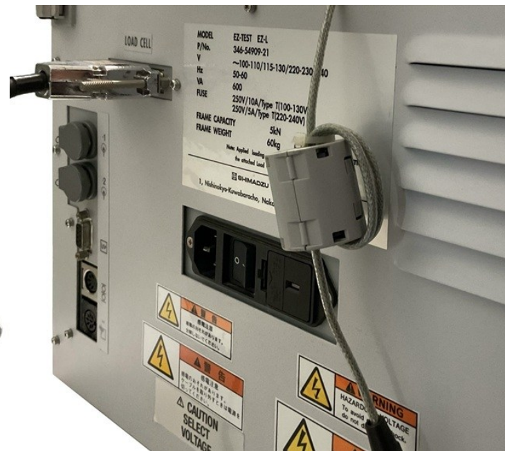
【装置背面】
