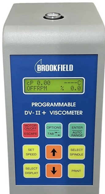
【装置拡大-2】
