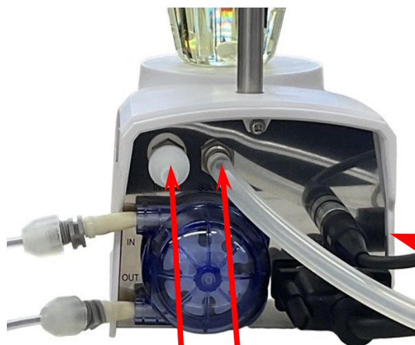
【自動給排水用ポンプ】
