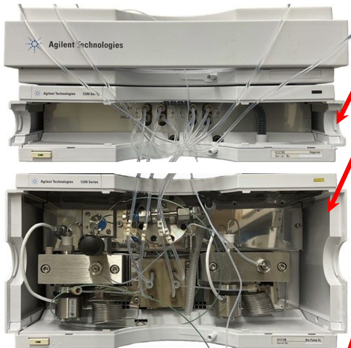
【デガッサとポンプ内部】
