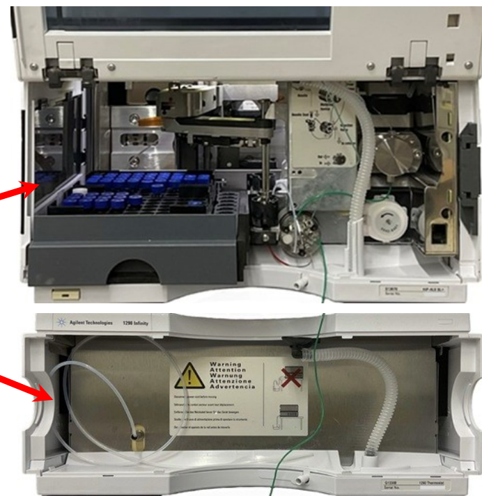
【オートサンプラーと冷却モジュール内部】
