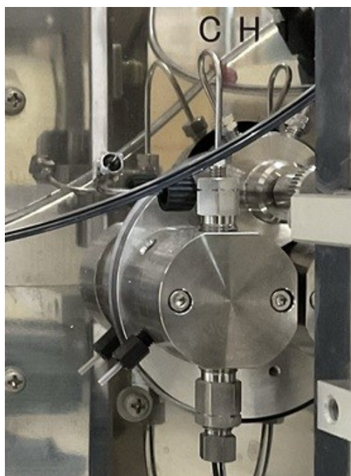
【ポンプ拡大】
