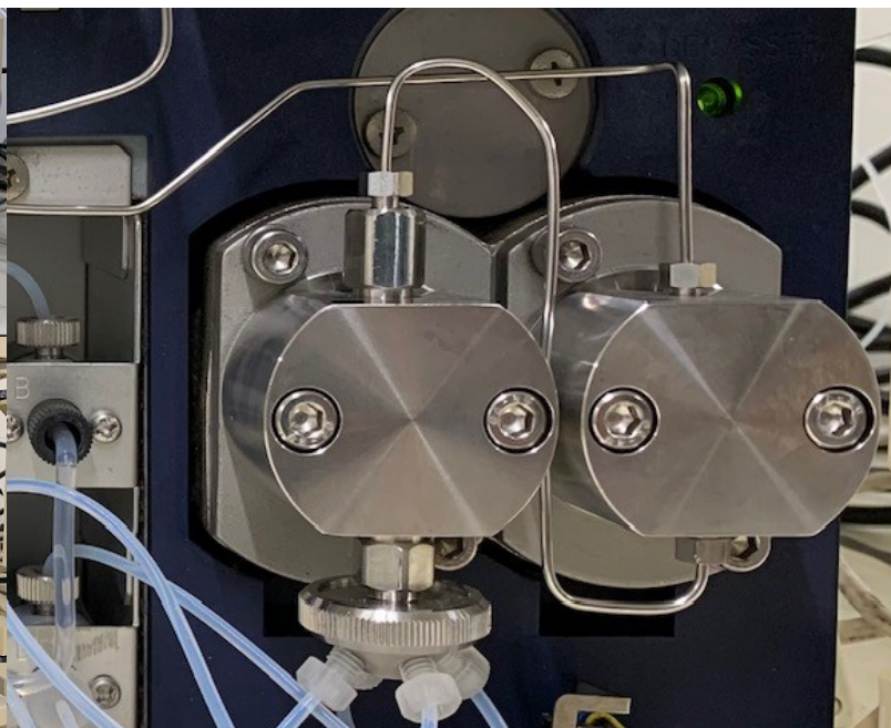
【ポンプ拡大】
