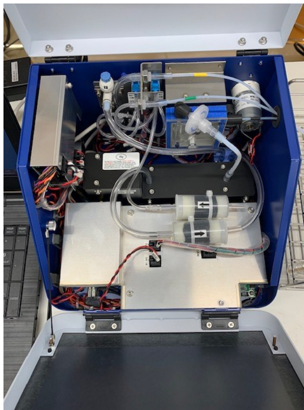
【装置内部】
