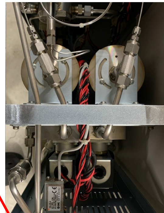
【装置内部上面から】
