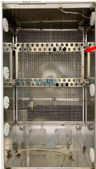
【カラムオーブン内部】
