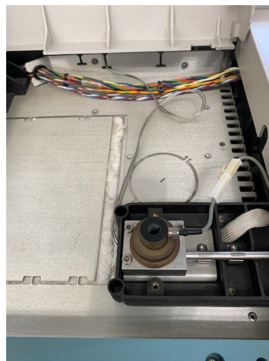
【検出器拡大】
