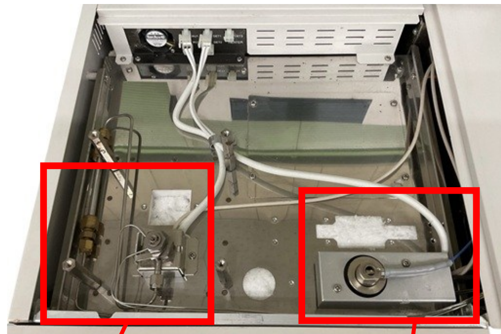
【FID検出器拡大】
