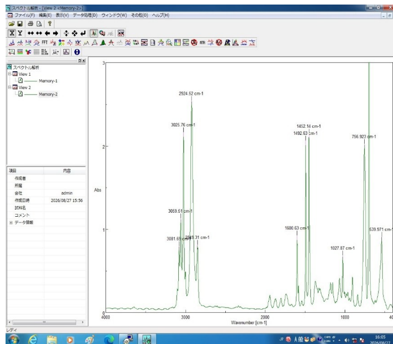
【FT-IR装置PS-FILM透過法測定後解析例-1,2】
